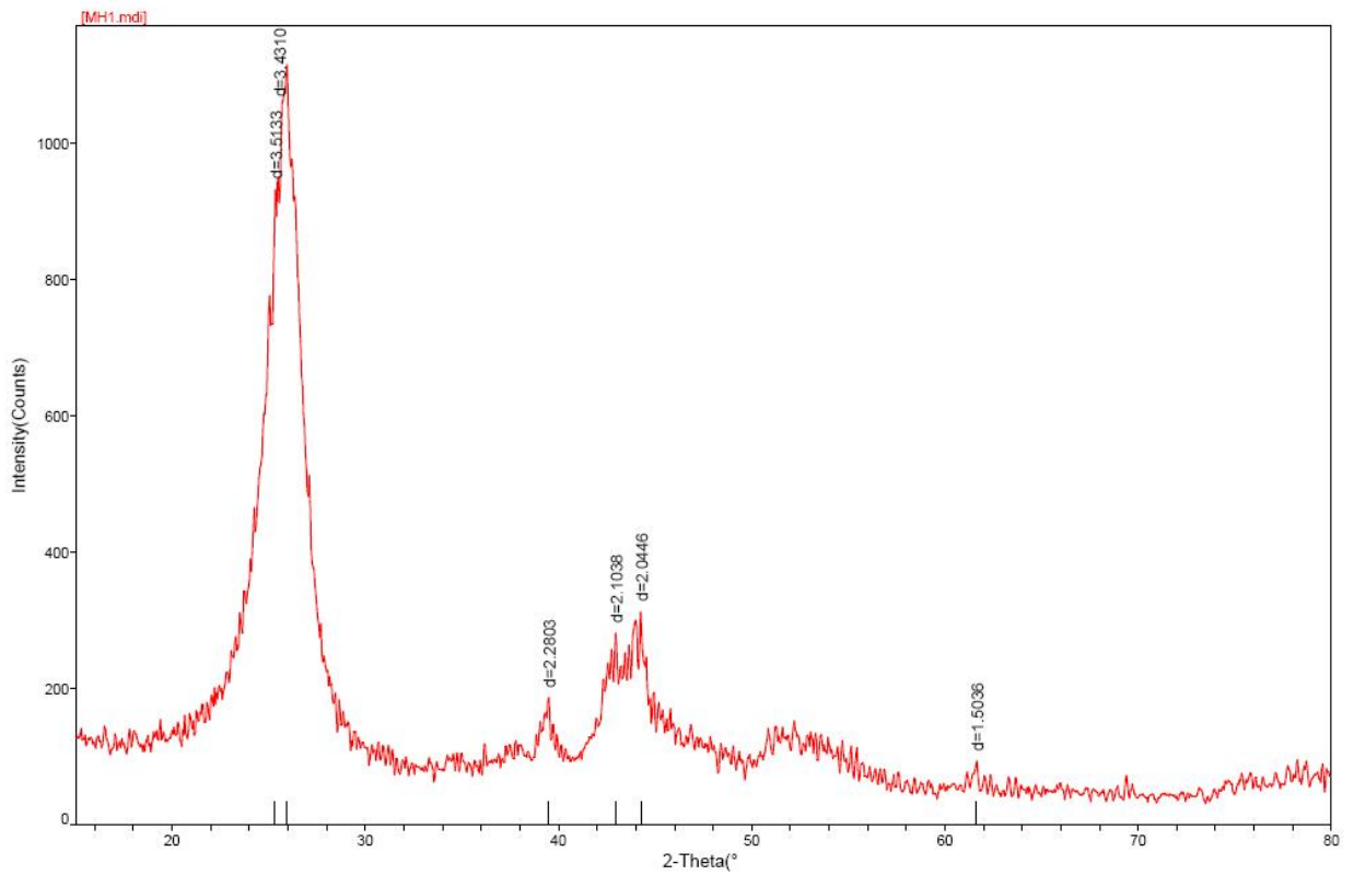
XRD
